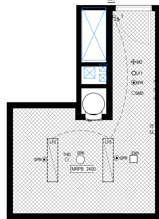
8 RCP-SLUICE Scale 1 : 50
